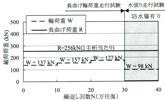
図-2 T荷重階段載荷試験
