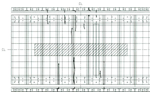
図-8 負曲げ荷重初期載荷 (T荷重階段載荷試験)
