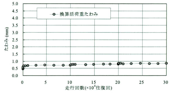
図-11 L荷重階段載荷試験の床版たわみ変化
