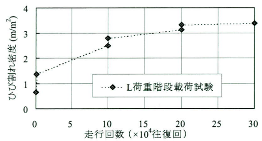
図-15 L荷重階段載荷試験のひび割れ密度の変化
