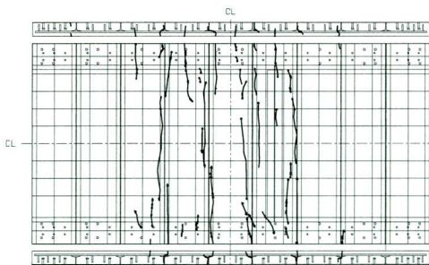
図-9 30万往復回終了 (T荷重階段載荷試験)
