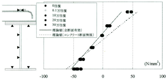
図-7 T荷重階段載荷試験の主桁系応力分布
