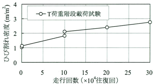
図-10 T荷重階段載荷試験のひび割れ密度の変化
