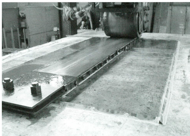
写真-3 水張り走行試験 (防水層無し)
