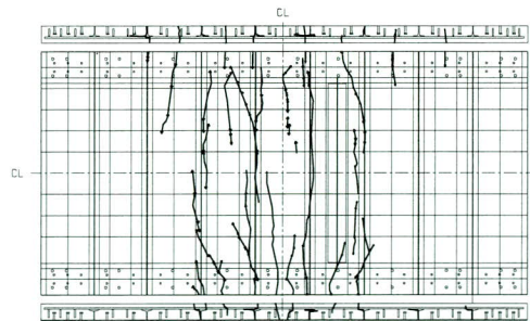
図-14 30万往復回終了 (L荷重階段載荷試験)
