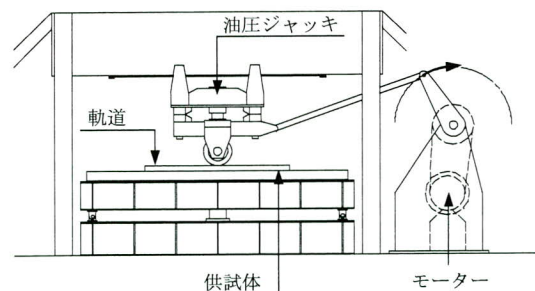
図-4 試験装置概要
