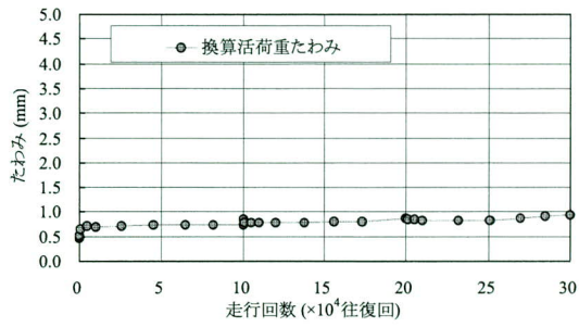
図-6 T荷重階段載荷試験の床版たわみ変化
