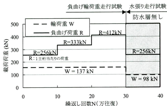
図-3 L荷重階段載荷試験
