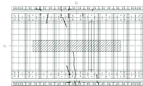
図-13 負曲げ荷重初期載荷 (L荷重階段載荷試験)
